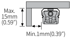
Min.1mm(0.39")
